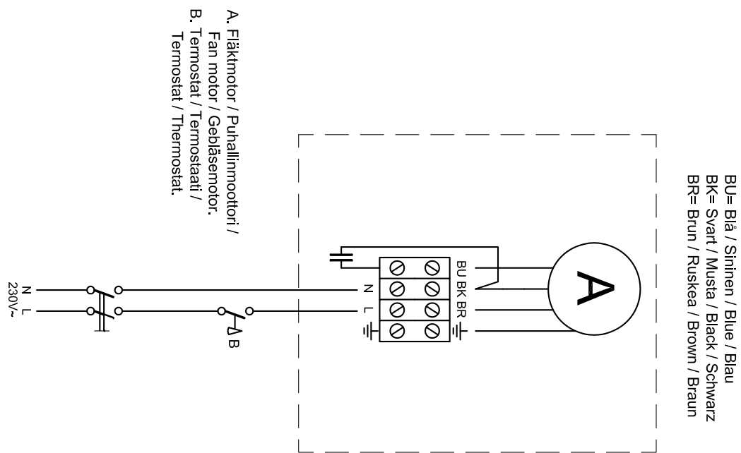
Kopplingschema / Sähkökaavio / Wiring diagram / Schaltplan
